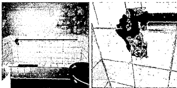
Foto 15: Sustitución de llaves y tubo en meninjerío.
